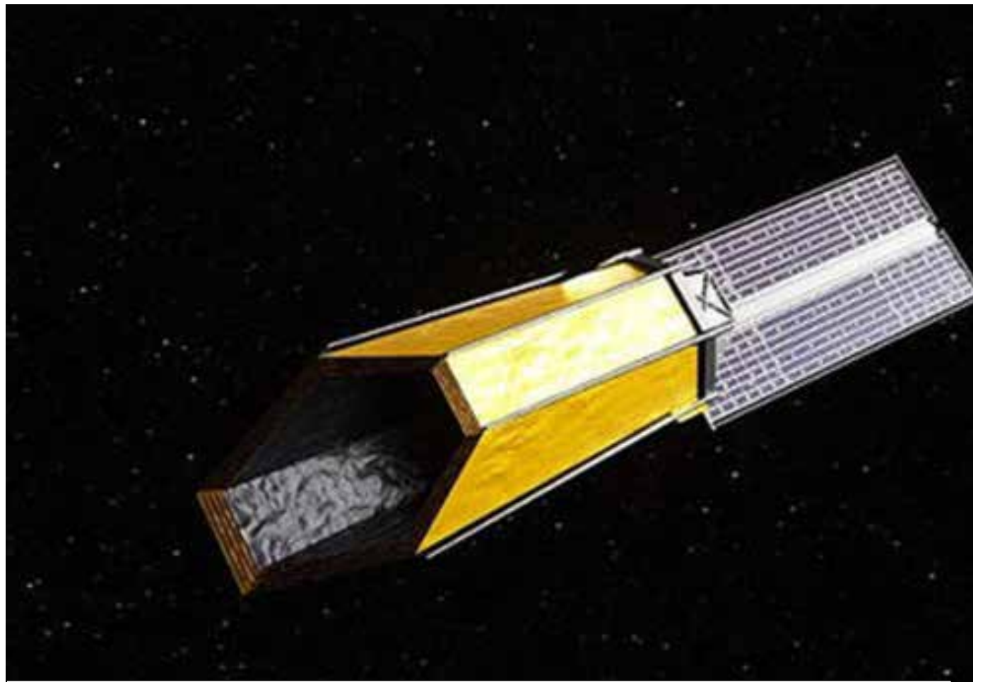
Astrofizikani Jessie Christiansen, i cili punon me NASA-n në kërkimin e ekzoplaneteve të ngjashme me Tokën, ka thënë se teleskopi i ri i planifikuar i agjencisë hapësinore amerikane, Observatori ‘Habitable Worlds’ (koncepti më lart), mund të gjejë prova të jetës aliene ‘në jetën tonë’
